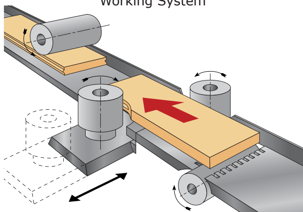
SCHEMA DI LAVORAZIONE Working System
