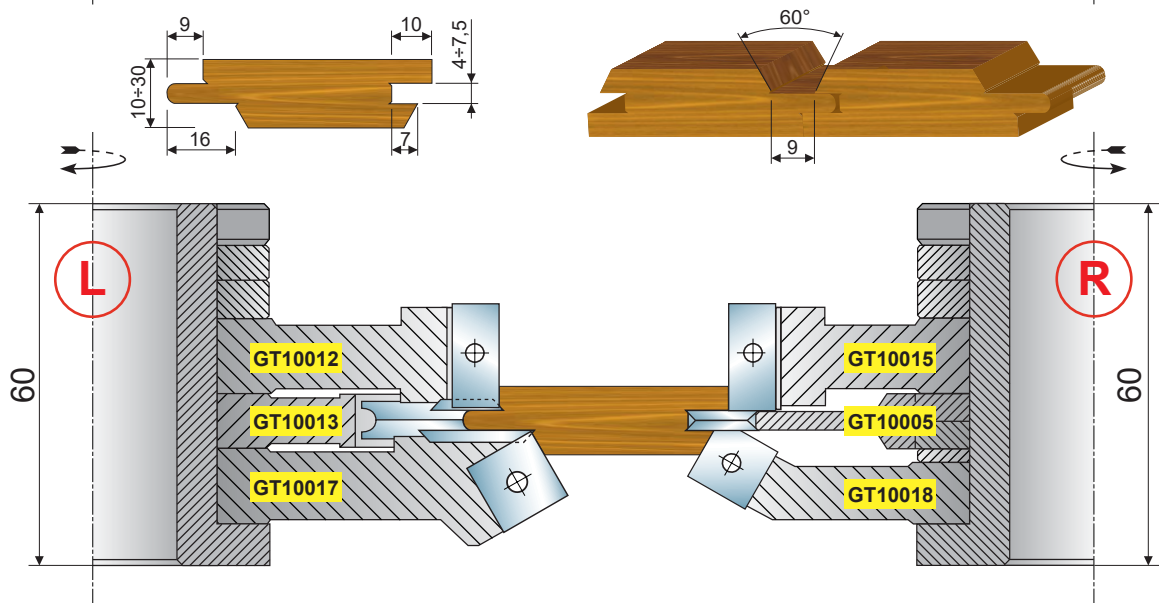
GRUPPO 6 Cutterhead set 6
