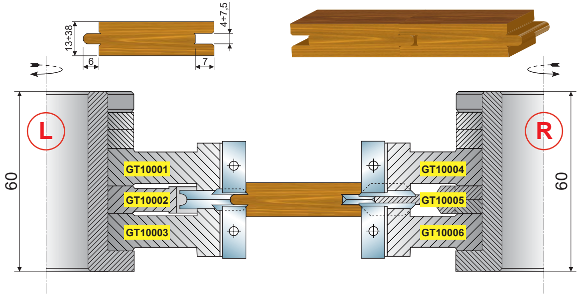
GRUPPO 1 Cutterhead set 1
