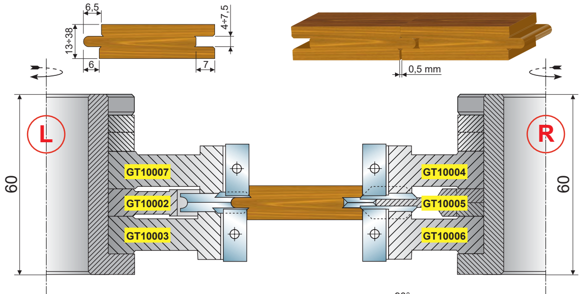
GRUPPO 2 Cutterhead set 2
