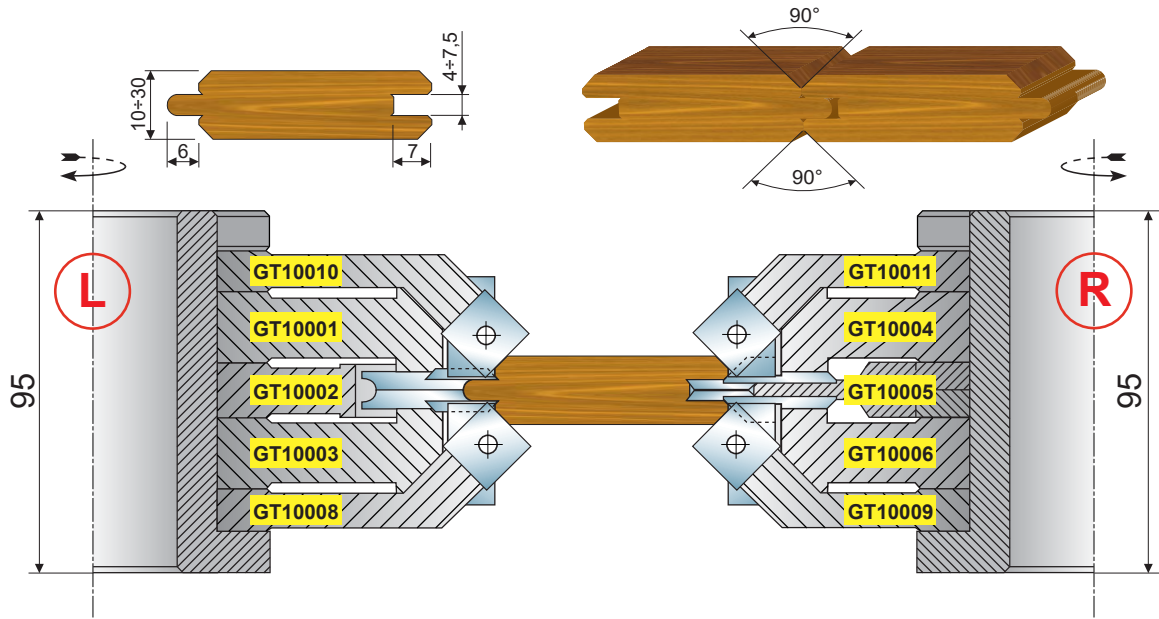
GRUPPO 4 Cutterhead set 4
