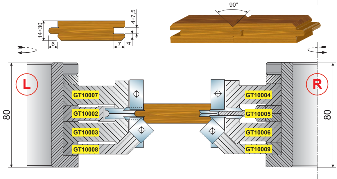
GRUPPO 3 Cutterhead set 3
