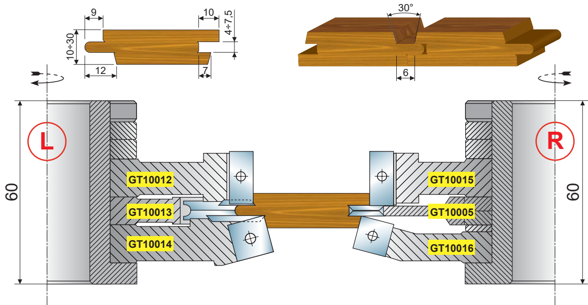
GRUPPO 5 Cutterhead set 5
