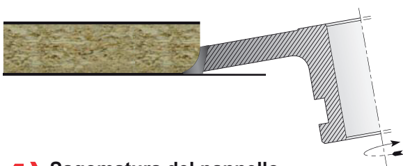
4) Sagomatura del pannello Panel profiling
