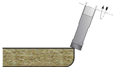
7) Refilatura superiore del bordo Edge's upper trimming
