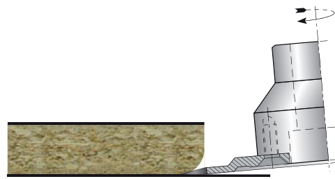
5) Incisione inferiore Lower engraving
