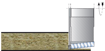
2) Sgrossatura del materiale in eccesso Exceeding material roughing
